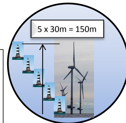
Comparaison du phare de la Banche, avec une éolienne marine de la taille du prototype qui sera installé au Carnet face à la centrale électrique de Cordemais (44)
